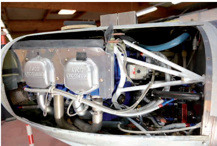
Le Lycoming de 180 ch est équipé du system christen (alimentation en huile) pour le vol sur le dos.
